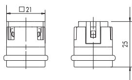
Штепсель EBM05CF00 Male Insert
